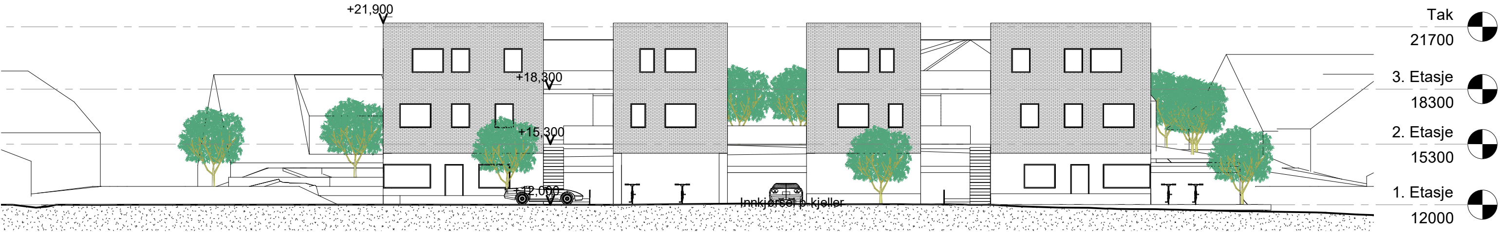
Oppriss sør 1 : 200
