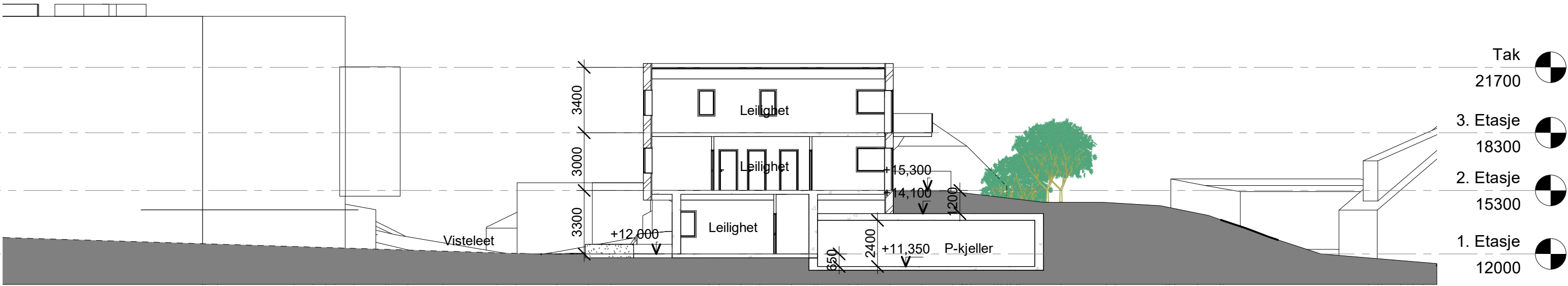
Snitt A 1 : 200
